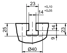
● B 部詳圖，比例3:1 ● B Block, Scale 3:1
